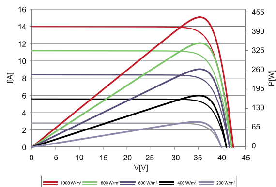
CHARAKTERYSTYKA PRĄDOWO-NAPIĘCIOWA
