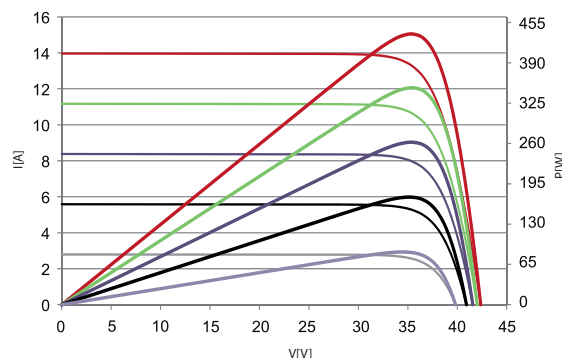
CHARAKTERYSTYKA PRĄDOWO-NAPIĘCIOWA
