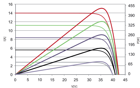
CHARAKTERYSTYKA PRĄDOWO-NAPIĘCIOWA
